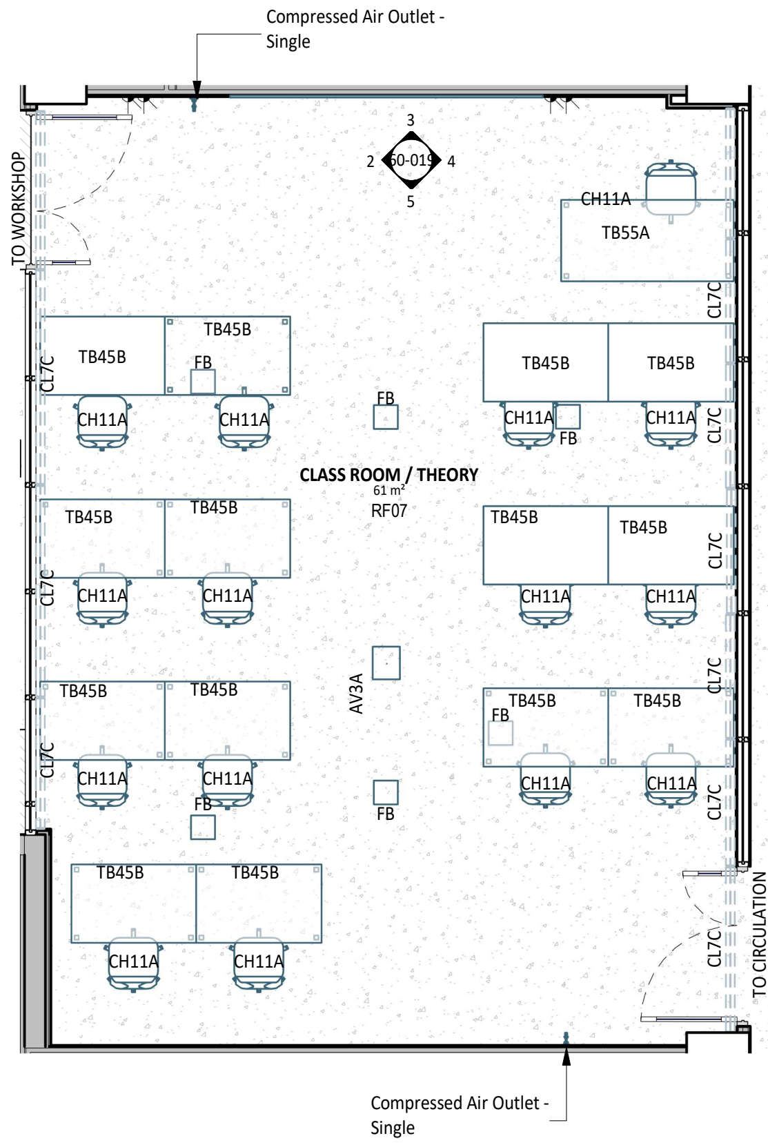
1 PLAN DETAIL 30-01 1 : 50
